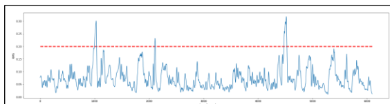
Рис. 9. Визуализация громкости цифрового сигнала тестовой записи с визуализацией порога детектирования высокого уровня интенсивности сигнала
